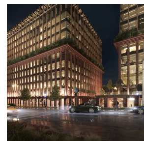
Топ-уровень архитектуры
