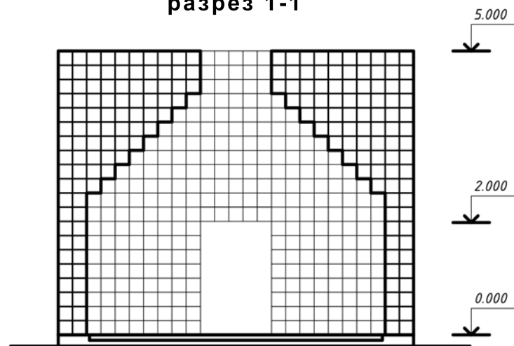
разрез 1-1
