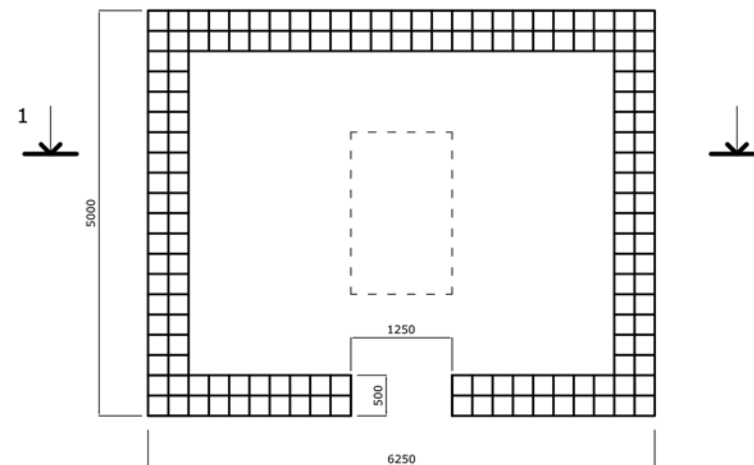
план
